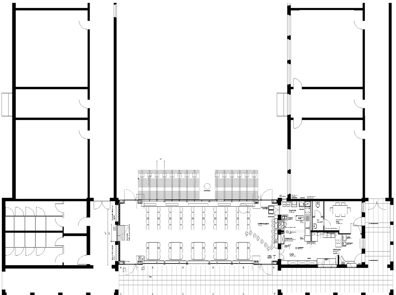
Grundriss
