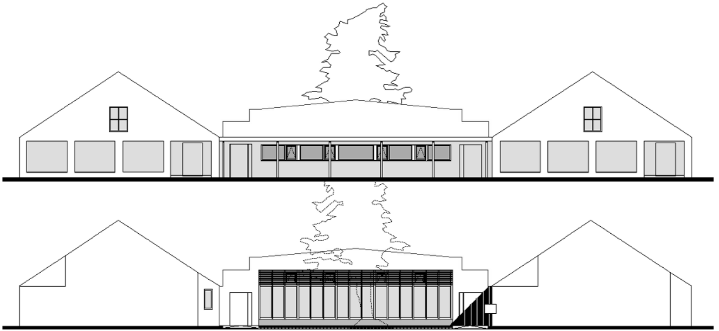
Ansichten
